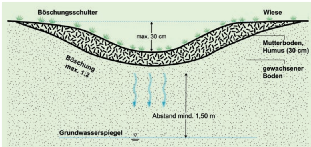
Abbildung 5: Muldenversickerung
