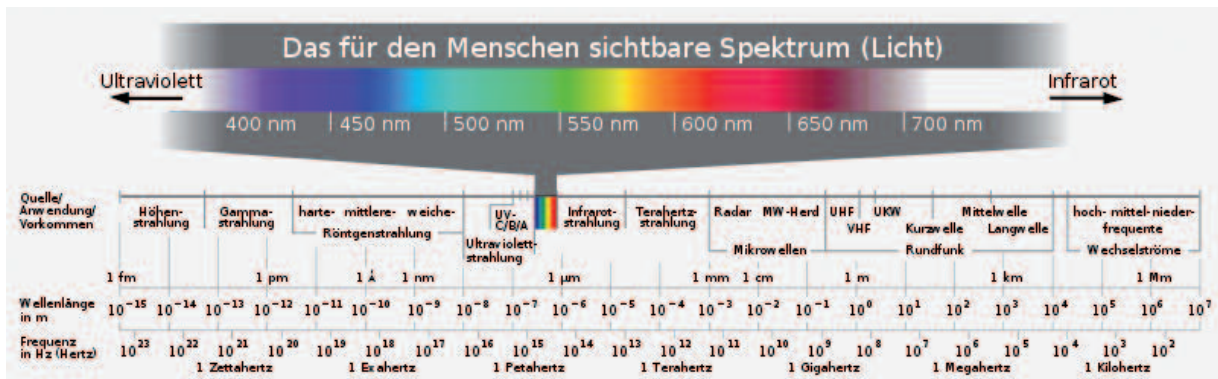
Abb. 2: Sichtbares Spektrum
