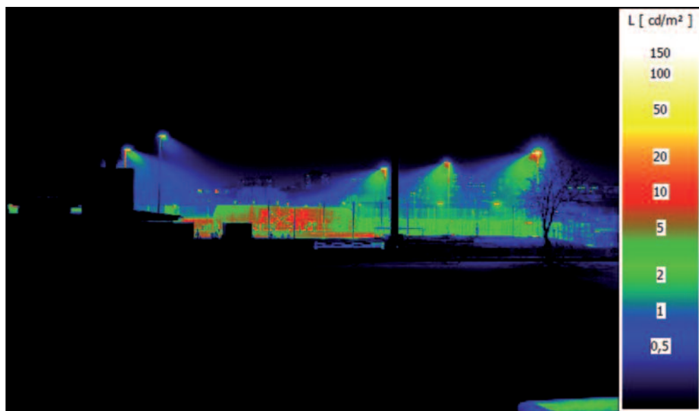
Abb. 41: Beispiel einer optimierten Trainingsplatz-Beleuchtung (Leuchtdichtemessung in Falschfarbendarstellung)
